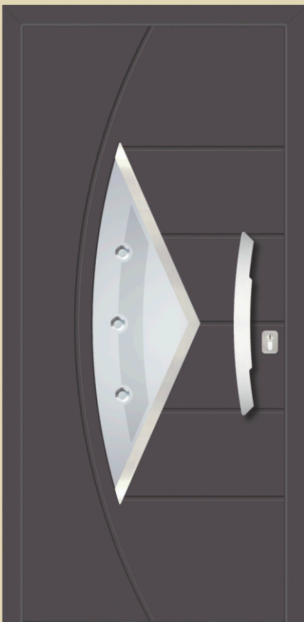
Aussenplatte AL grigio antico Innenplatte AL grigio antico Glas DPB - Sandgestrahltes "Satinato" Glas mit geklebtes Fazettenglas Aplikation INXC-externe Griff GPS 590h Rosette RKP 50
