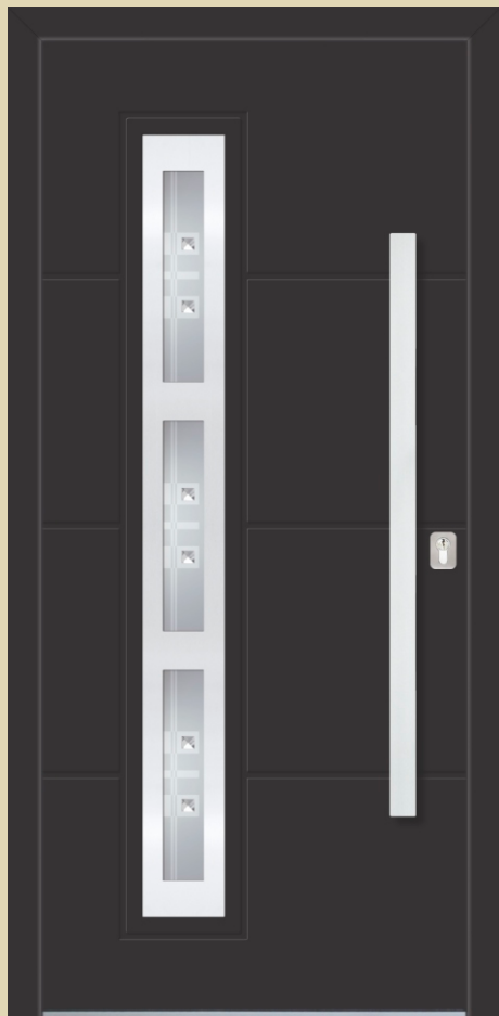
vanjska ploča AL 7016 mat unutrašnja ploča AL 7016 mat staklo DPB - pjeskareni satinato s bijelim fazetama aplikacija INXC-vanjski rukohvat DPS 115h rozeta RKP 50
